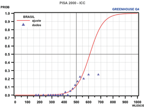
Figura 7. Curva característica do item (ICC) para a questão Efeito Estufa 4, dentre os alunos brasileiros, na prova de Ciências do Pisa 2000; no eixo horizontal, o escore dos estudantes, e no vertical, a probabilidade de acerto na questão
